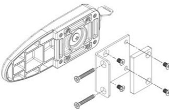
Montage sur le battant de la porte
