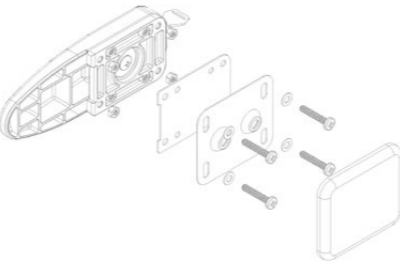
Montage à travers la paroi
