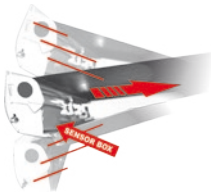
Wind-Detection System: sensore del vento
