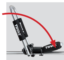
Funzione basculante Hull-a-Port Pro 837 può essere ripiegato contro la barra portatutto quando non viene utilizzato per ridurre la resistenza al vento e l'ingombro.
