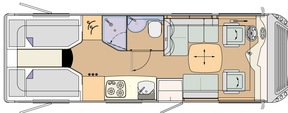
CARVER 742 L 7480 x 2380 x 3190 mm
