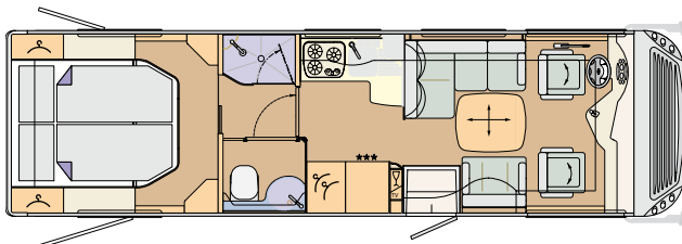
CHARISMA 841M Iveco Daily: 8480 x 2380 x 3290 mm, MAN: 8620 x 2380 x 3460 mm
