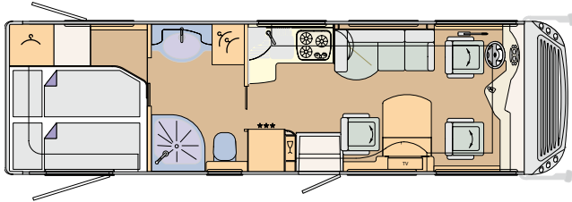
CHARISMA 840F Iveco Daily: 8480 x 2380 x 3290 mm, MAN: 8620 x 2380 x 3460 mm
