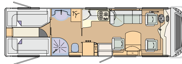
CHARISMA 840L Iveco Daily: 8480 x 2380 x 3290 mm, MAN: 8620 x 2380 x 3460 mm
