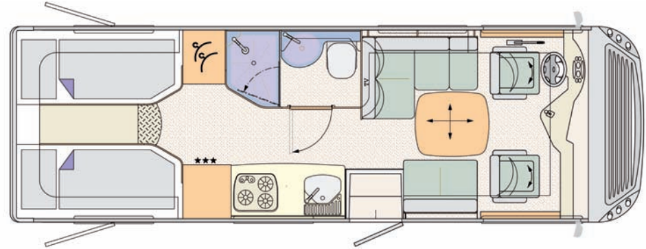
CARVER 742 L 7480 x 2380 x 3190 mm
