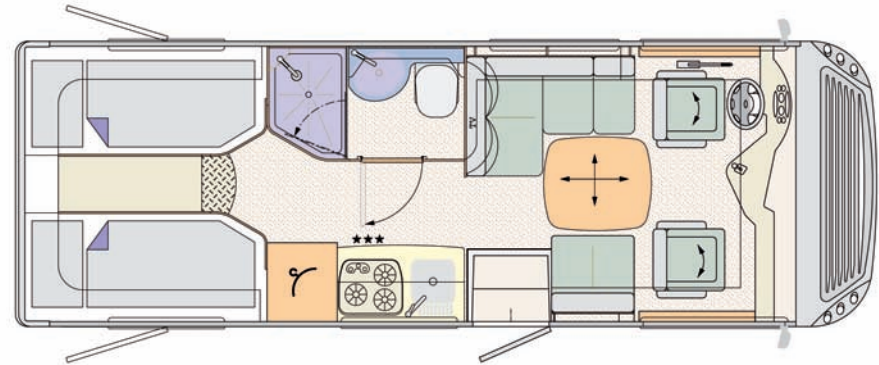
CARVER 692 L 6980 x 2380 x 3190 mm
