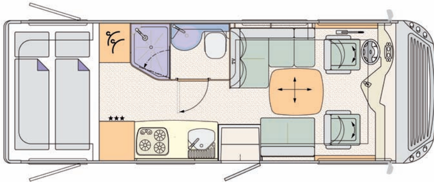
CARVER 692 H 6980 x 2380 x 3190 mm
