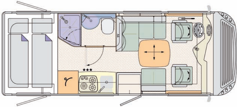
CARVER 642 H 6480 x 2380 x 3190 mm
