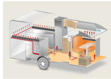
Riscaldamento nella cellula abitativa Il sistema di riscaldamento garantisce una distribuzione ottimale del calore in tutto l'ambiente.
