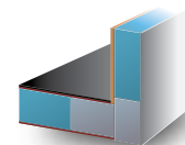
Struttura priva di legno con isolamento XPS
