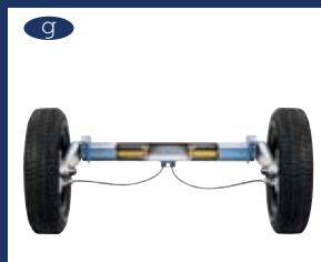
Essieu freiné ALKO équipé de suspensions à torsion caoutchouc | ALKO Independent Rubber Suspension (IRS) axle
