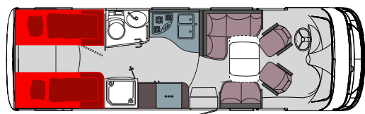
I 7900 GD
