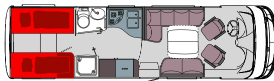
I 8400 GD
