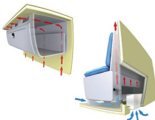
Schema di principio di funzionamento del sistema di riscaldamento ALDE. Non corrisponde alla descrizione precisa del prodotto e/o del mobilio.
