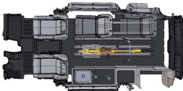
3-4 posti viaggio e biciclette
