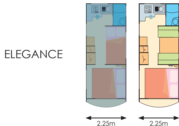
LM400CB2 Cuisine en Bout 4 places
