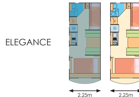
LM490CE Chambre enfant 6 places
