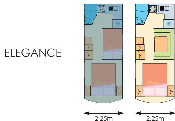
LM490CB Cuisine en Bout 4 places (lits jumeaux en option)
