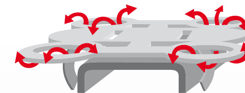
Lastverteilung durch bewegliche Tellerfedern
