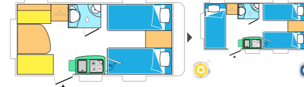
ANTARES 450 + PACK STYLE 450 / 4,70 x 2,15 m
