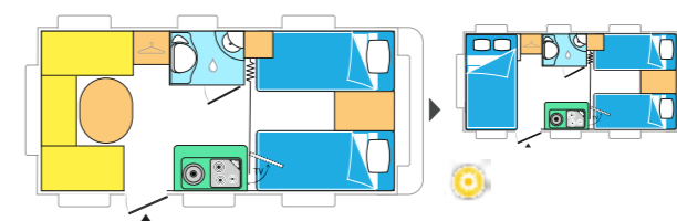
ALLEGRA 450 / 5,00 x 2,15 m
