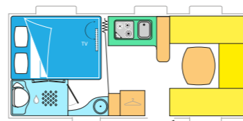
ALLEGRA 420 / 4,20 x 2,15 m
