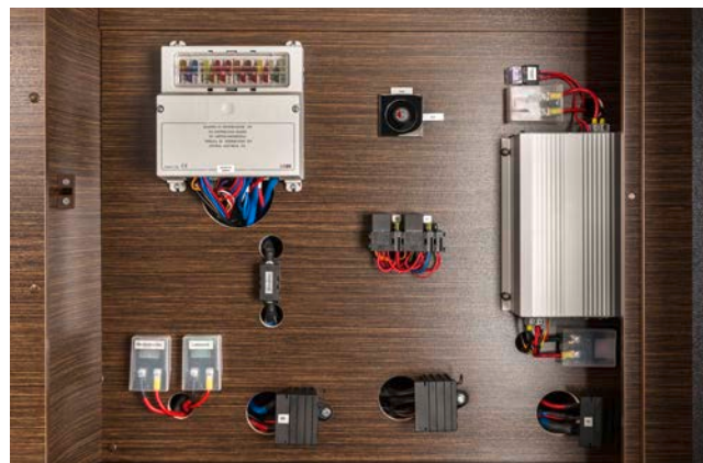
BATTERIE-MANAGEMENT-SYSTEM
