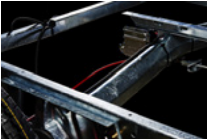
Extra vridstyvt chassi. Extra balkar mellan längsgående chassireglar ger stabilare golv och extra vridstyvt chassi. Mellanbalkar för bästa stabilitet. Chassit har utliggare från längsgående sidobalk för att avlasta från tyngden där golv och vägg är sammanfogade. Karossen tål mycket hög belastning, till exempel när stora mängder snö ligger på taket.
