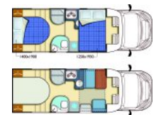
BARON 581
