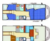
BARON 53G
