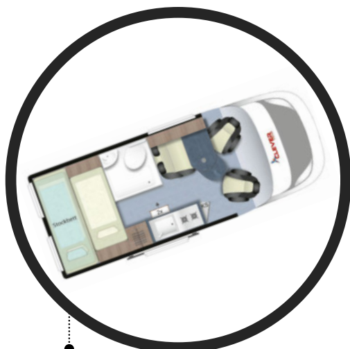
Grundriss für 3 Personen
