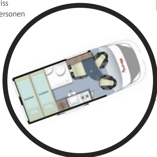
Grundriss für 4 Personen
