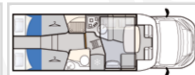
BARON 573 ← l. 7410 mm →
