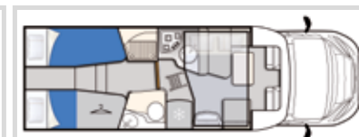
T-LOFT 530 ← l. 7410 mm →
