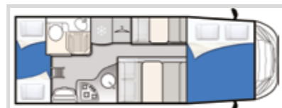
BARON 22 ← l. 6990 mm →
