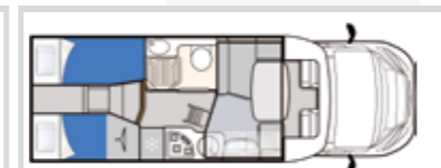
BARON 565 ← l. 6990 mm →
