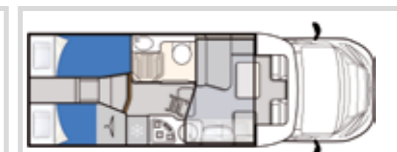
T-LOFT 529 ← l. 6990 mm →
