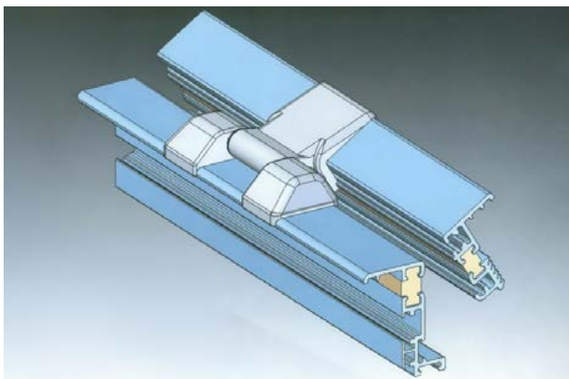
THERMISCH GETRENNTER KLAPPENRAHMEN
