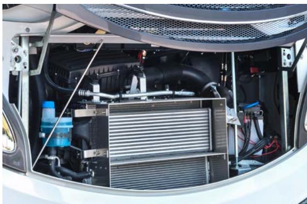
MOTORRAUM
