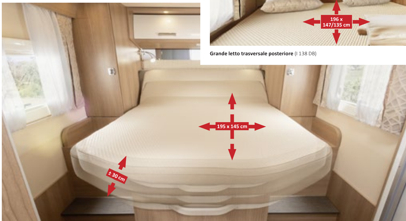
Con richiesta di brevetto: superficie del letto traslabile di 30 cm per passare comodamente da posizione giorno a posizione notte (I 144 QB)
