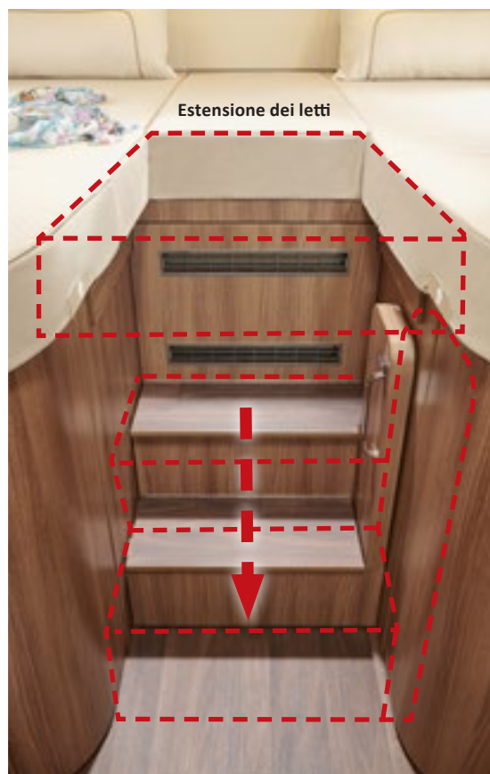
Estensione dei letti Gradino estraibile per accedere ai letti (con richiesta di brevetto), per un comodo accesso anche usando la prolunga dei letti, in tutte le posizioni gli armadi guardaroba sono raggiungibili dall'alto
