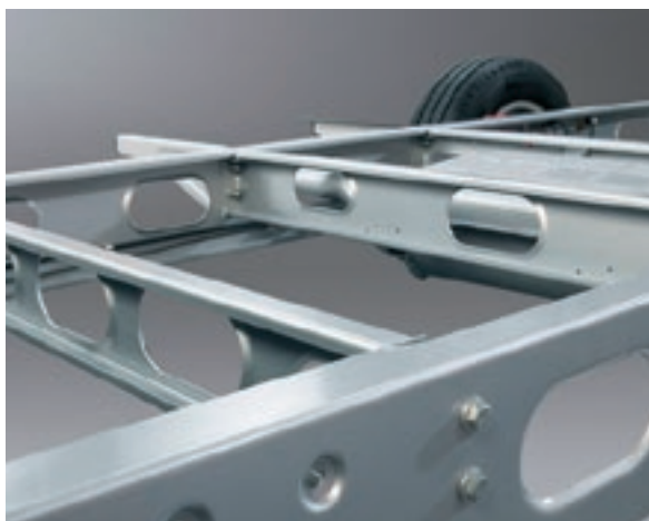
Telaio ribassato AL-KO speciale "light"
