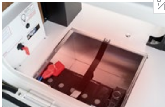
Vano batterie riscaldato con stacca batterie. Di serie: 2 batterie al gel da 80 Ah, facilmente raggiungibili, optional batteria al litio da 90 Ah con caricabatteria specifico elettronico.
