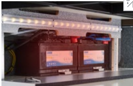
Centrale batterie di serie: 2 batterie al gel da 80 Ah nella cantina nel doppio pavimento riscaldato e stacca batterie, optional batteria al litio da 90 Ah con specifico caricabatteria elettronico
