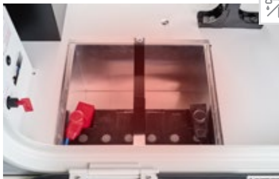
Centrale batterie riscaldata con stacca batterie; di serie: 1 batteria al gel da 80 Ah, ampliabile a 2 batterie da 80 Ah, optional batteria al litio da 90 Ah con specifico caricabatterie elettronico
