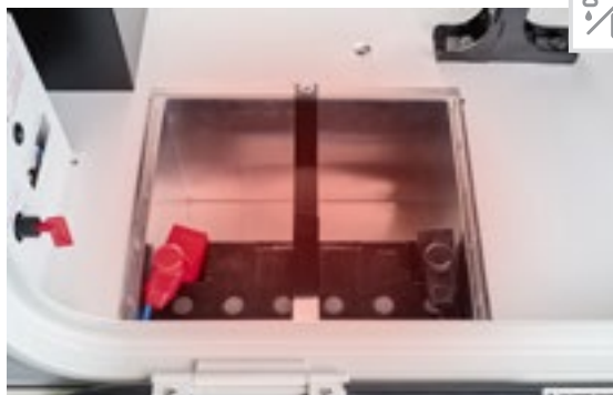
Vano batterie riscaldato con stacca batterie; di serie: 1 batteria al gel da 80 Ah, ampliabile a 2 batterie da 80 Ah, optional batteria al litio da 90 Ah con specifico caricabatterie elettronico
