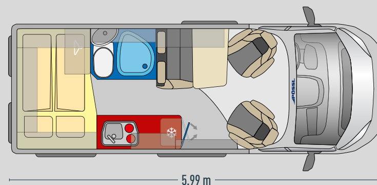
Grande dinette | via libero per quattro persone
