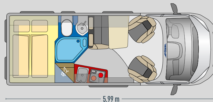
Area di seduta extra large | Passaggio comodo di quattro persone (opzionale, nuova forma del tavolo dal 2020)
