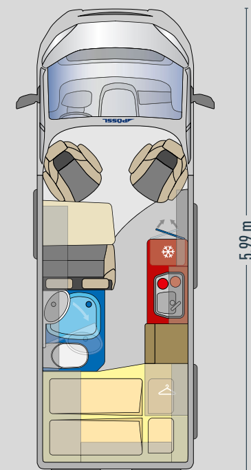
Area di seduta extra large | Con imbottitura sagomata ergonomica | Tavolo con unità girevole (opzionale) | AkyRoof regolabile con tettuccio illuminato (opzionale)
