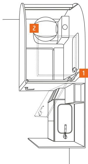
Bagno nella tipologia 450 FU
