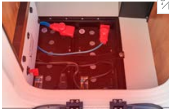
Centralina delle batterie riscaldata con interruttore di corrente; di serie: 2 batterie al gel da 80 Ah, in posizione facilmente accessibile, batteria al litio opzionale, 90 Ah con caricabatteria elettronico e touch-display separato.
