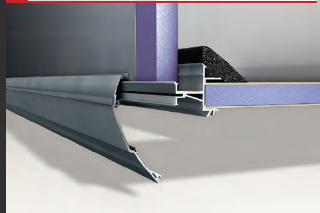
3 Collegamento parete laterale/pavimento con stabile longherone
