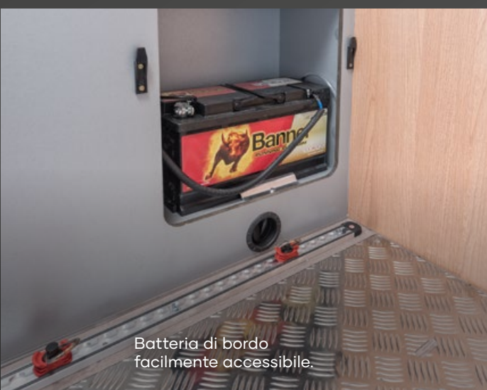
Facile accesso all'impianto elettrico di bordo.
