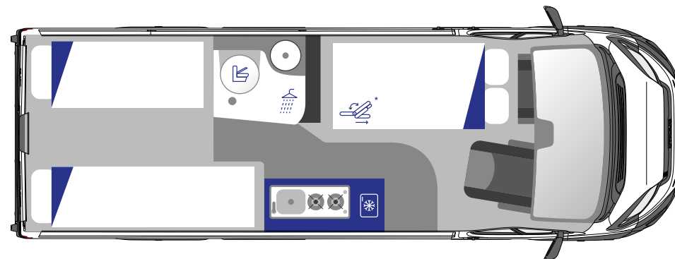
Night plan
