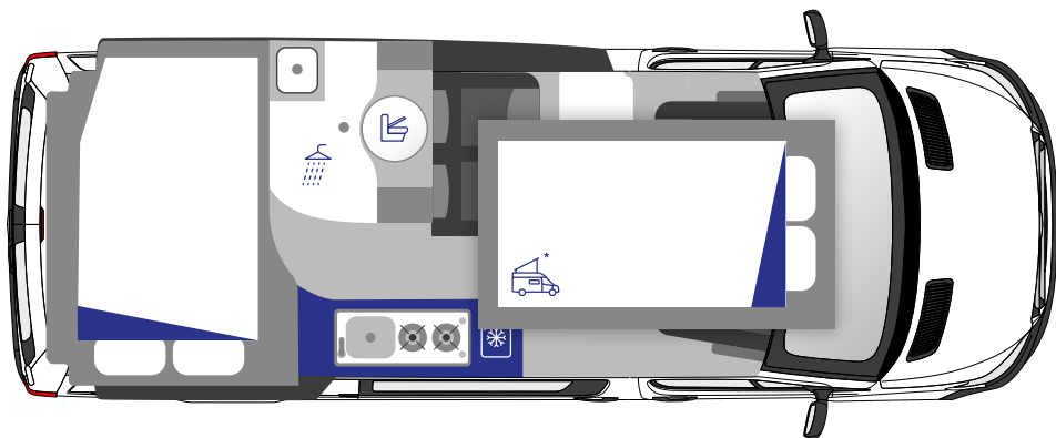
Night plan
