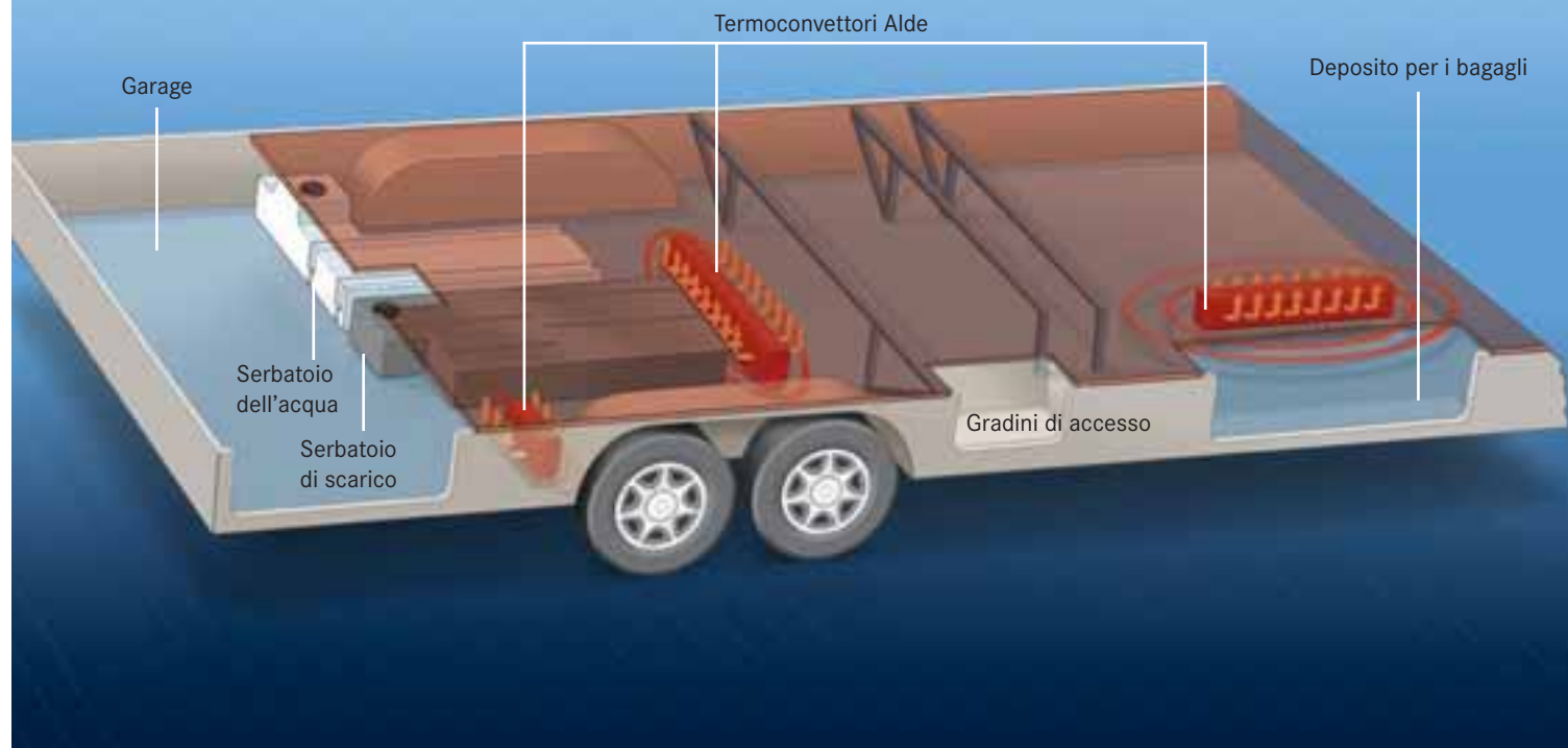
Circolazione del riscaldamento ad acqua calda Alde
