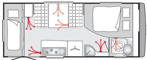
Riscaldamento di interni Truma - Ripartizione ad aria calda
