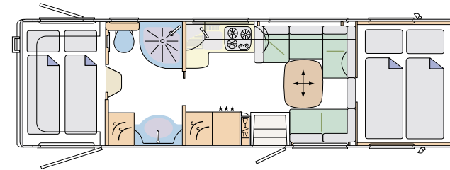
Cruiser C1 840 HR mit Premiumbad
