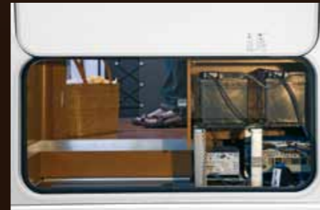
Von außen zugängliche Versorgungseinheit mit heizungsnah liegenden AGM-Batterien (95 Ah)
