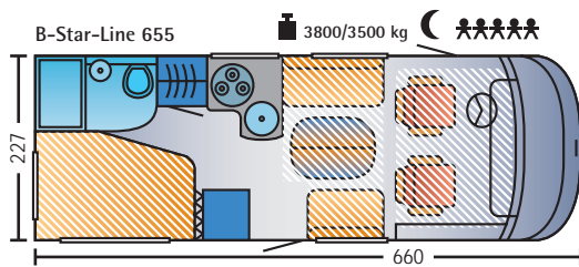
Längssitzgruppe/Französisches Bett
