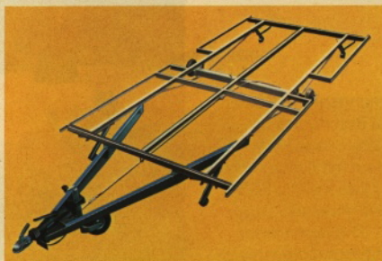
Stabiles Ganzstahlchassis mit verzinkter Deichselgruppe und Drehstützen.
