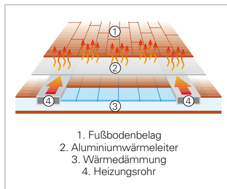
Fußbodentemperierung (Option)
