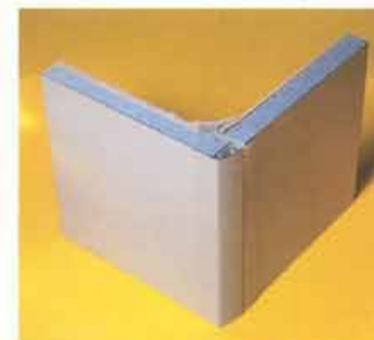
Die Flair-Ringanker-Wandverbindung 35 mm starke Dach- und Seitenwände aus Aluminium (außen 1 mm - innen 0,8 mm) dazwischen Styrofoam
