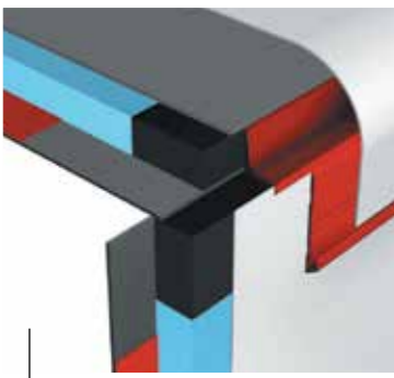
Roof and side walls connected by aluminium profiles Taket och sidoväggarna förenade med aluminiumprofiler
