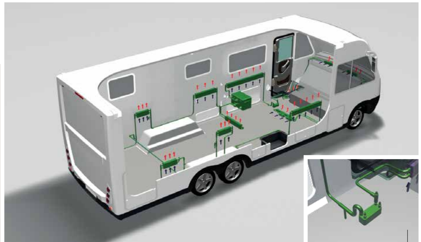
Thermal exchanger Värmväxlare
