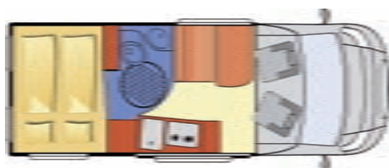
► Pianta: 2Win Style
