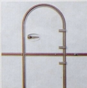
Geteilte Tür mit verdeckt verschraubten massiven Türbändern und Türfeststeller. Alle Beschläge und Leisten korrosionsgeschützt eloxiert.
