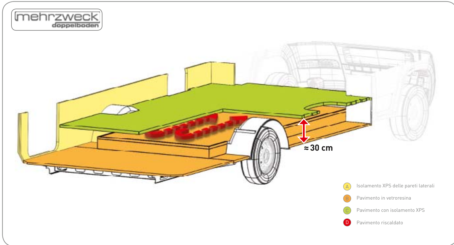
Il doppio pavimento multifunzionale Knaus dei modelli Sun TI e Sky i.
